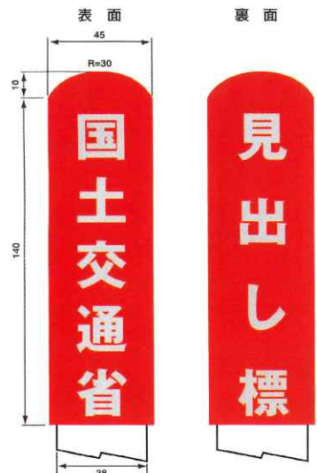
■ ポールの頭部 (単位mm)
