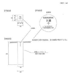
図一〇 札幌市基準点 (3級) 標準設置図
